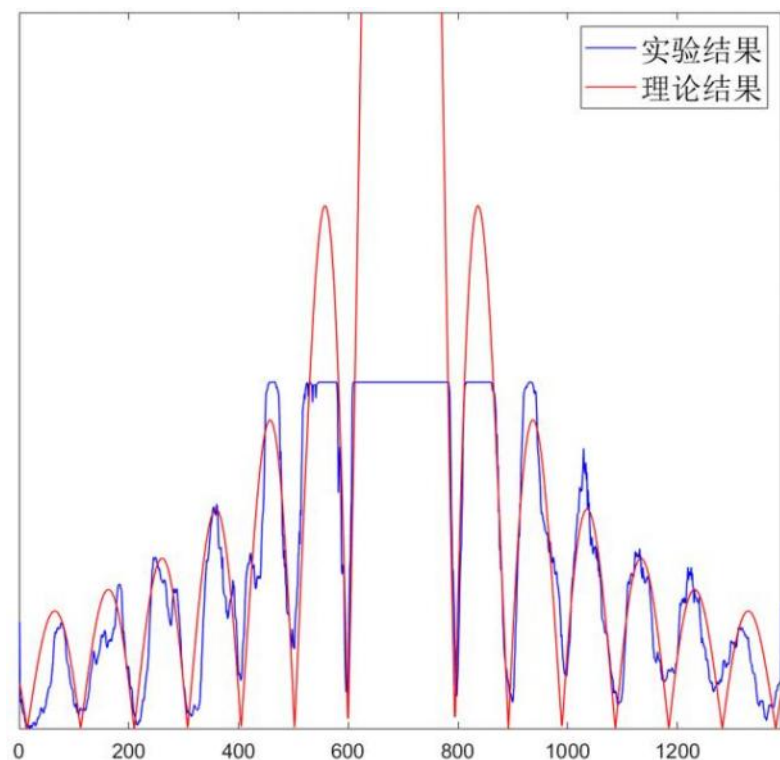
图27 正方形夫琅禾费衍射水平轴光强分布(边长 300\mu m )
